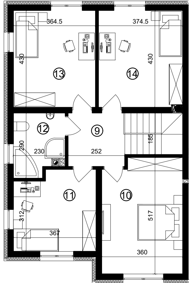
ZESTAWIENIE POWIERZCHNI PIĘTRO - LOKAL 1
