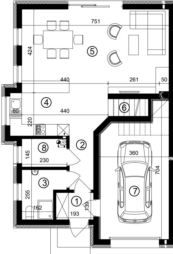
ZESTAWIENIE POWIERZCHNI PARTER - LOKAL 1
